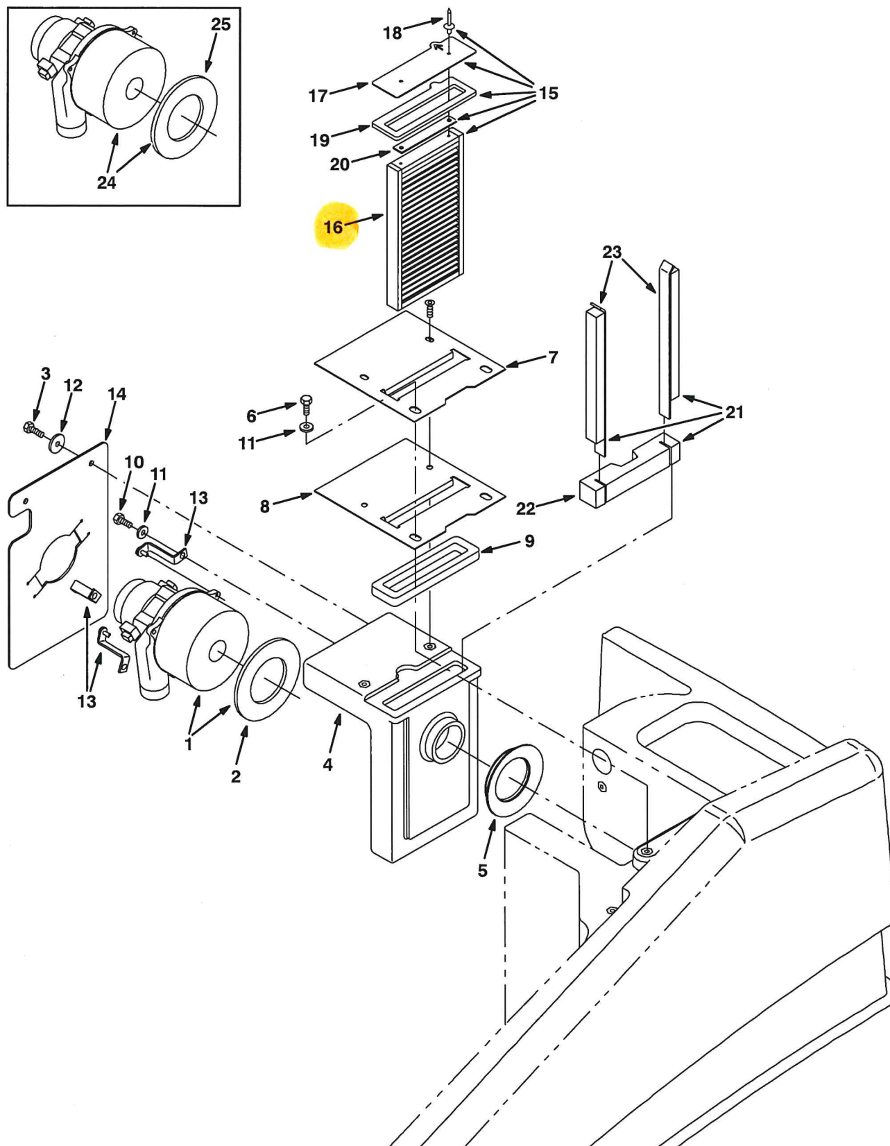
Fig. 19 - Vacuum Fan Kit, Single — Vakuumgebläse-Satz, Einfach — Lot extracteur, simple
