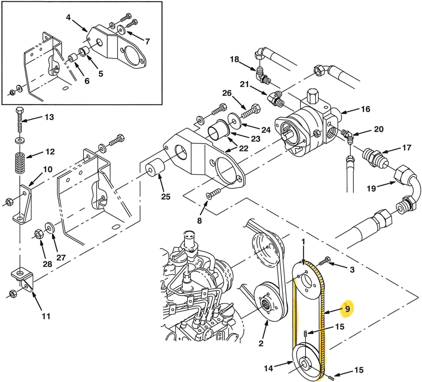
Fig. 52 - Hydraulic Belt Drive Pump Group — Riemenantrieb-der-Hydraulikpumpe — Groupe Pompe hydraulique d'entraînement de courroie
