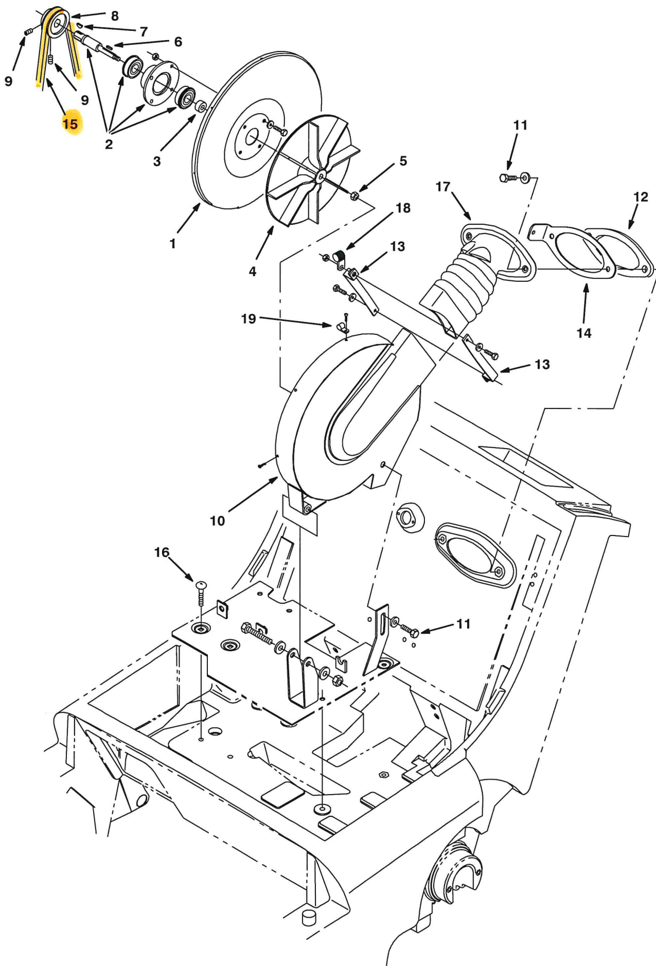
Fig. 8 - Vacuum Fan Group Vakuumbelüftung-Gruppe Groupe extracteur
