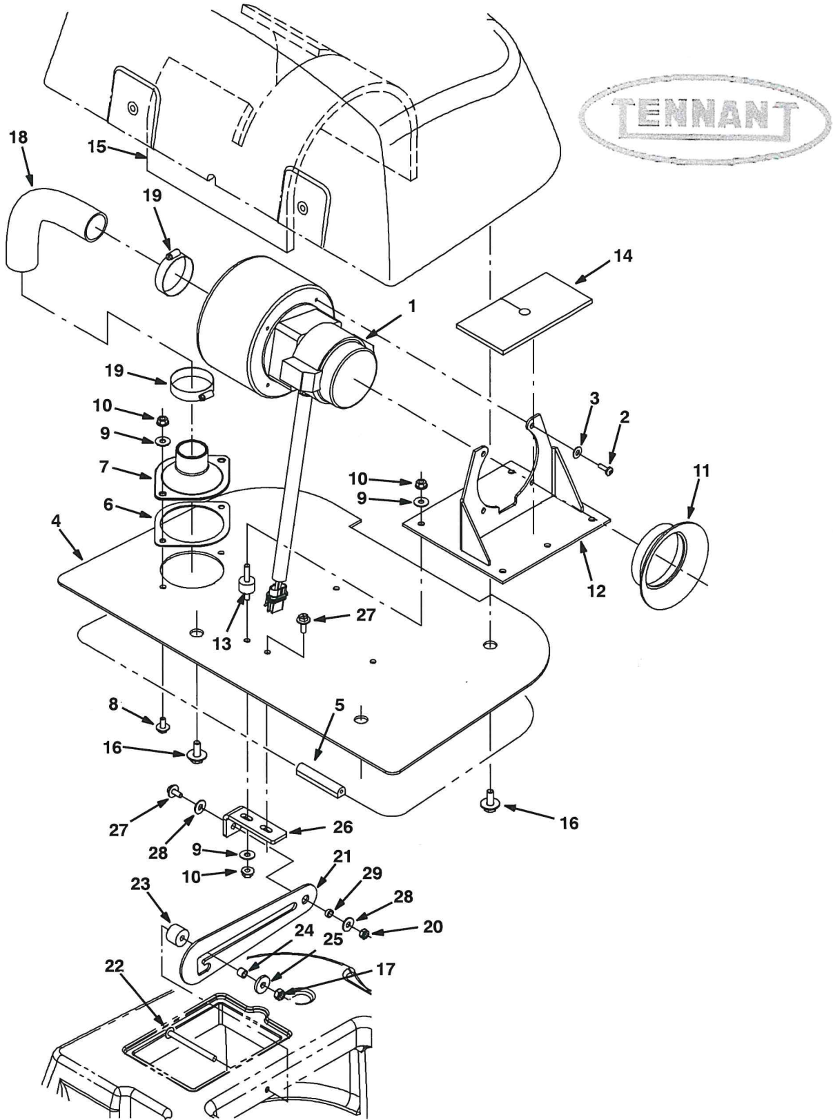
Fig. 23 - Vacuum Fan Group
